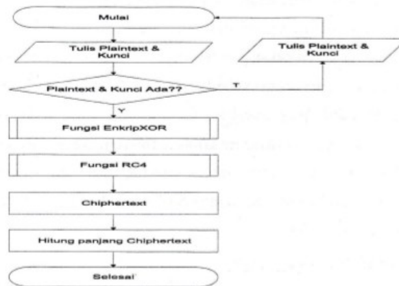
Gambar 4. Diagram Alir Program Enkripsi
