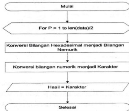
Gambar 8. Diagram Alir Fungsi DeskripXOR
