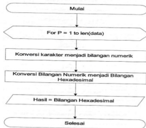
Gambar 7. Diagram Alir Fungsi Enkrip XOR
