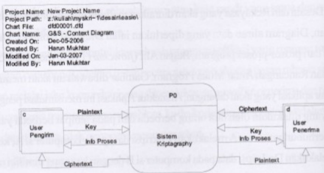
Gambar 2. Diagram Konteks
