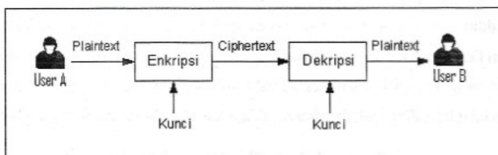
Gambar 1. Arsitektur Sistem
